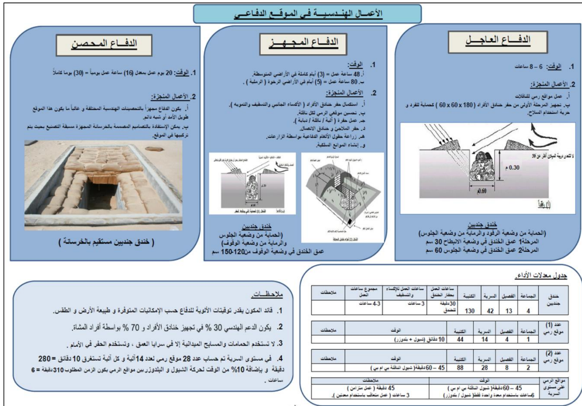
الشكل رقم (1) الأعمال الهندسية في الموقع الدفاعي
